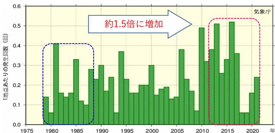
図1 北海道地方のアメダス1地点あたりの1時間降水量30mm以上の年間発生回数
