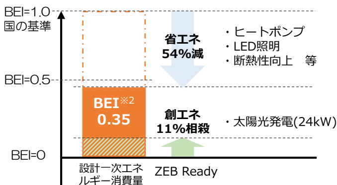
ZEBの概念図
