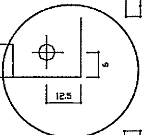
底板取付図 S=1/1
