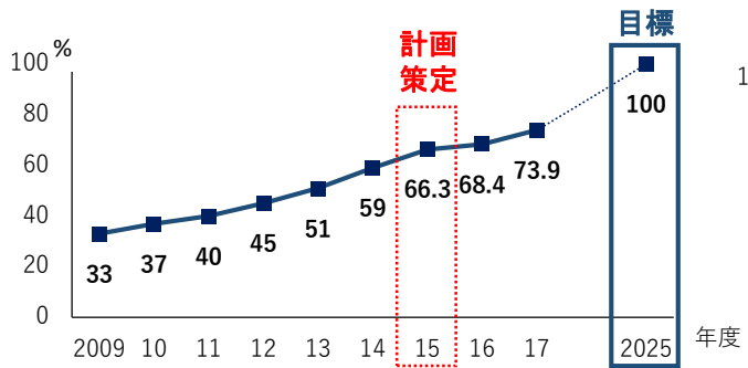
緊急輸送道路上等の橋梁の耐震化率(道道)の推移
